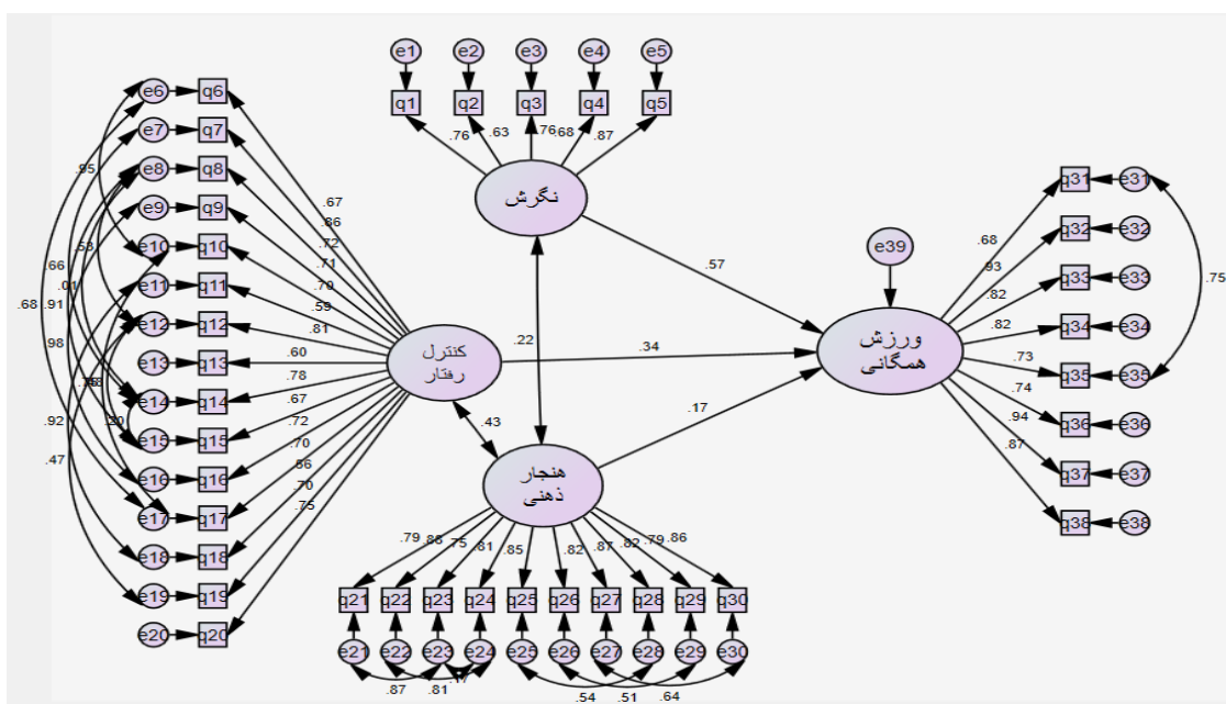
شکل ۲. مدل معادله ساختاری اصلاح شده پژوهش
