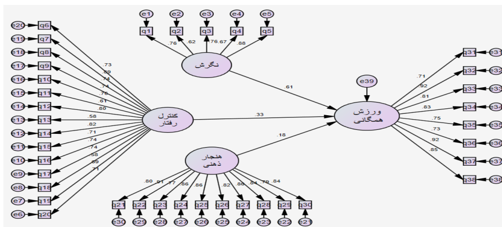
شکل ۱. مدل معادله ساختاری پژوهش
